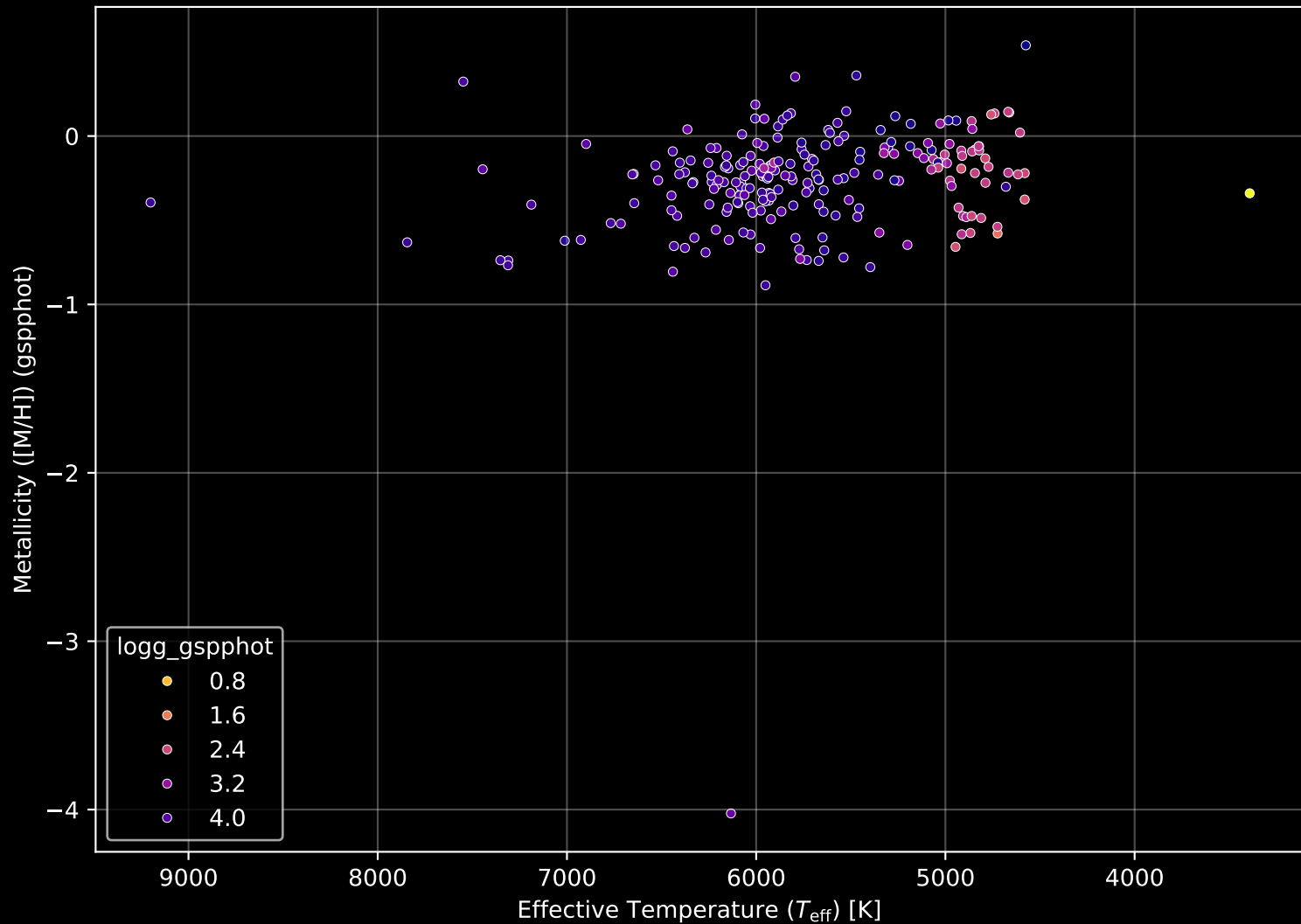
GALAH DR4 Field: [7160] Stellar Population Parameters (n= 224)
