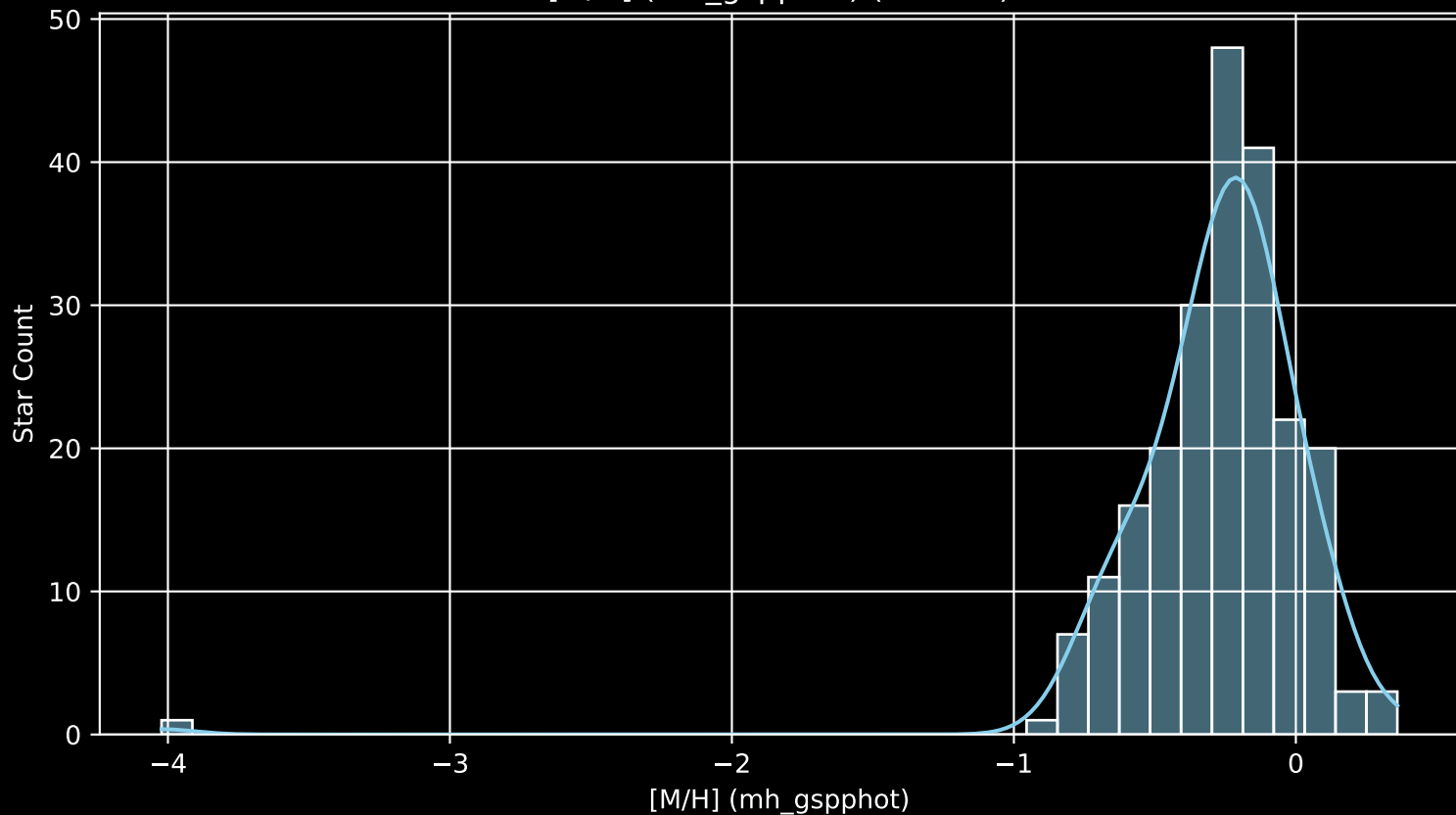
GALAH DR4 Field: [7160] [M/H] (mh_gspphot) (n= 223)
