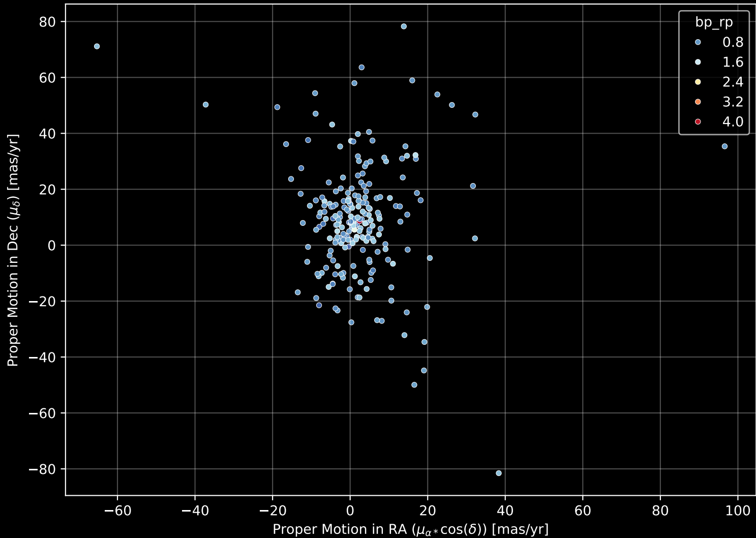
GALAH DR4 Field: [7160] Proper Motion Diagram (n= 224)
