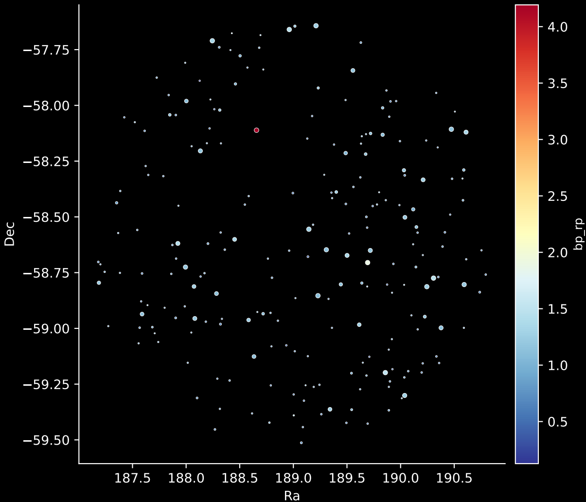
GALAH DR4 Field: [7160] Stars: 224
