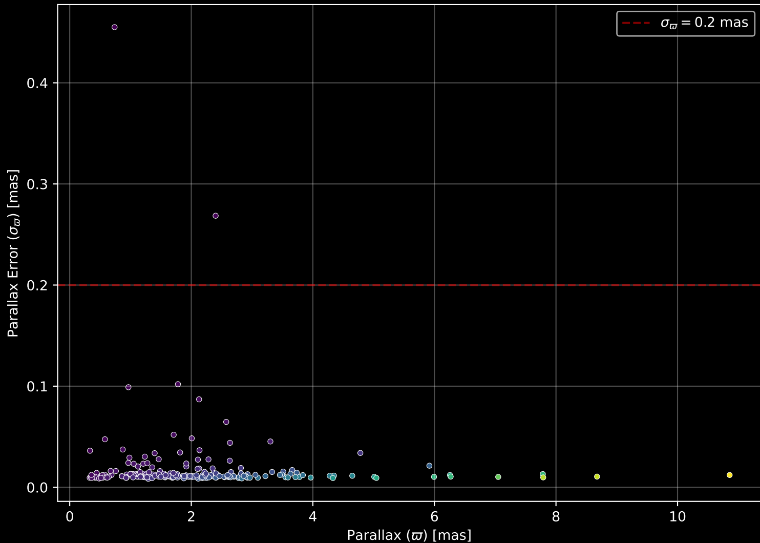
GALAH DR4 Field: [7160] Parallax Quality (n= 224)
